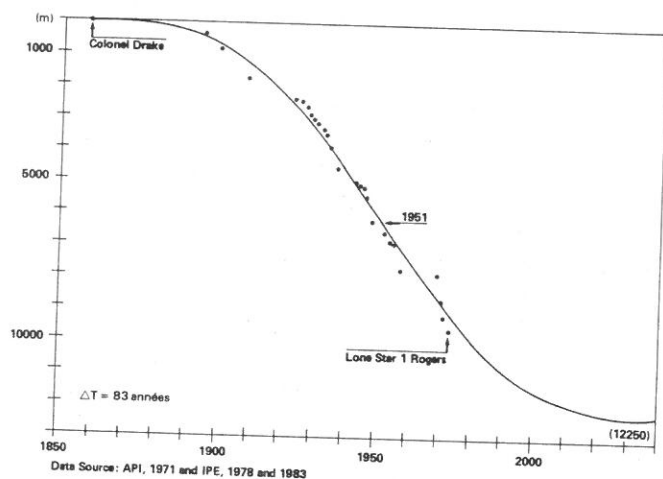
Fig. 8 Profondeur max. de forages d'exploration aux E.-U. avec courbe logistique en m. Source: Grubler et Nakicenovic, 1988.
