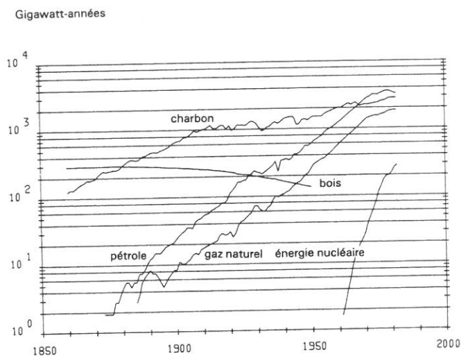
Fig. 2 Croissance de la consommation d'énergie primaire au niveau mondial en GW-années. Source: Grubler et Nakicenovic, 1988.
