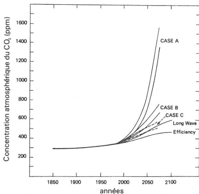
Fig. 14 Concentration atmosphérique du CO 2 dans différents scénarios d'approvisionnement d'énergie. Source: Ausubel et al., 1988.
