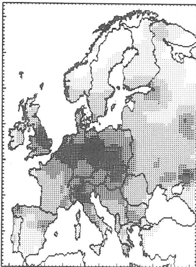
Fig. 12 Dépôt de soufre (en haut) et d'azote (en bas) des émissions d'Europe en 1980 (g/m 2 /an). Source: IIASA Transboundary Air Pollution Project, 1989.
