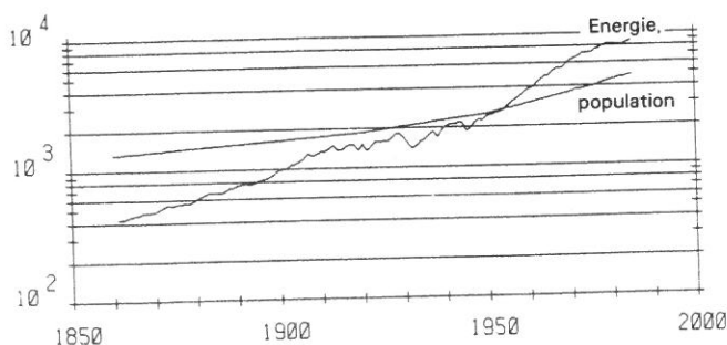
Fig. 1 Croissance de la population (Mio.) et de la consommation d'énergie (GW-années) (1 GW-année correspond à 1 mio. de t de charbon équivalent). Source: Nakicenovic et Gilli, 1989
