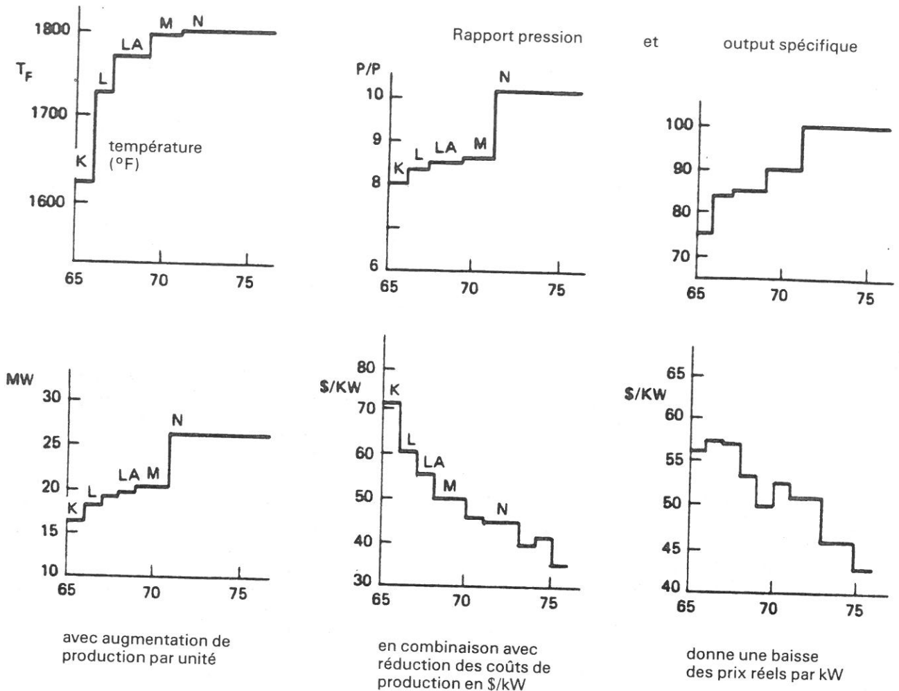
Fig. 9 Histoire technologique d'une turbine à gaz (MS 5001). Source: Lee, 1987.
