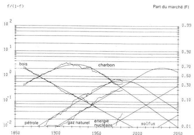
Fig. 3 Substitution des sources d'énergies primaires au niveau mondial; transformation F/(1-F) des parts de marché (F). Source: Marchetti et Nakicenovic, 1979 .
