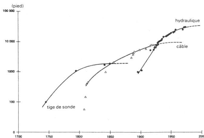
Fig. 7 Profondeur max. des technologies de forage (en pied). Source: Grübler et Nakicenovic, 1988.
