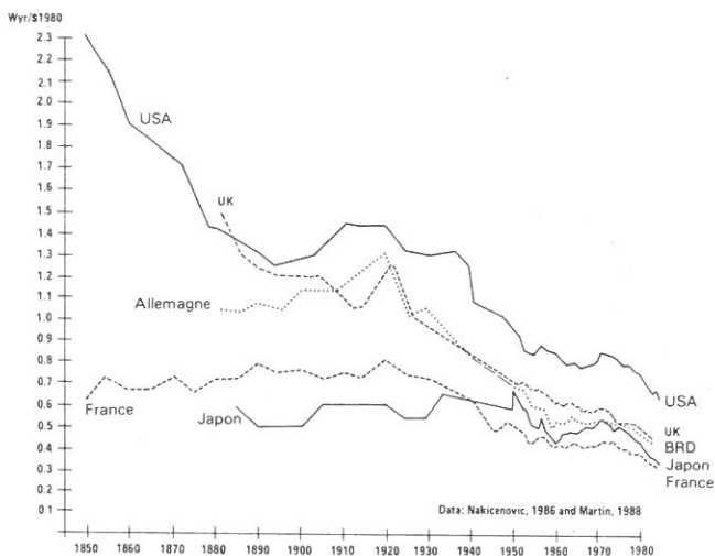
Fig. 10 Consommation d'énergie par unité du produit intérieur brut (en monnaie constante) y incluant des sources d'énergie non commerciales (bois) en Watt-année par $ 1980. Source: Nakicenovic et Gilli, 1989.
