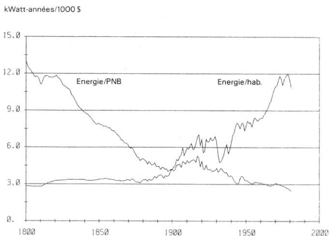
Fig. 11 Consommation d'énergie primaire (énergie commerciale, bois, foin, énergie hydraulique et éolienne) par unité du produit national brut (PNB) et consommation d'énergie par hab. aux E.-U. depuis 1800 en kWatt-année par 1000 $ (1958) PNB et par hab. Source: Nakicenovic, 1986.
