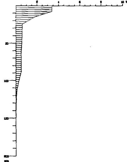
Solonchaks
